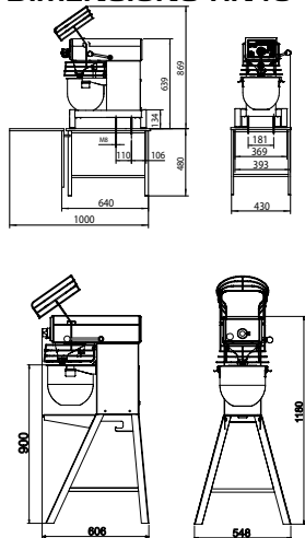
DIMENSIONS RN10
